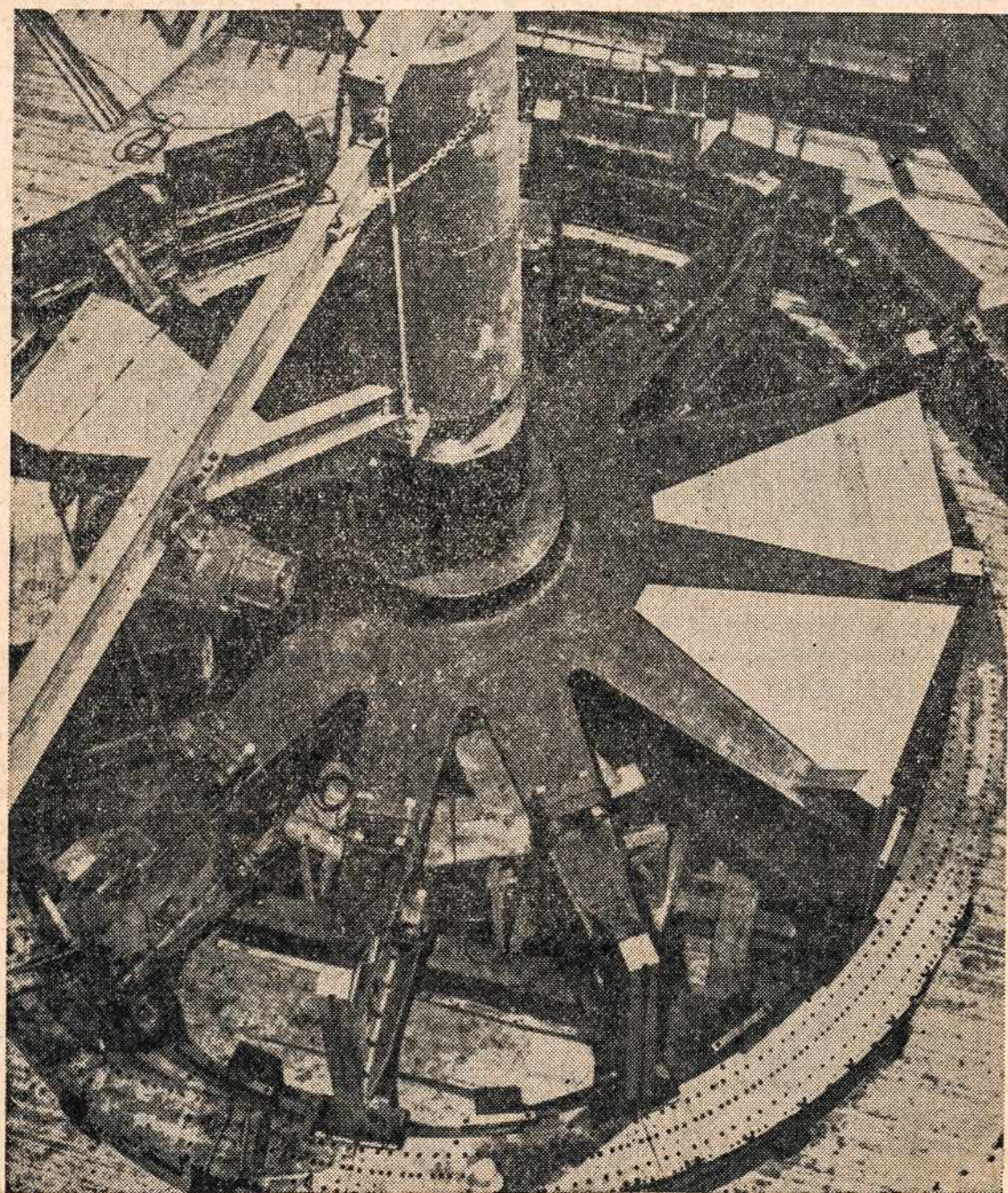
Vaižde matomas gamintuvus jėgos. Šis milžiniškas gamintuvus yra įtaisomas Grand Coulee Dam, Washington, upės Columbia tvenkiny, kuris turi 100 mylių vario vielos ir galės gaminti 108,000 kilowattų ir yra 24 pėdų aukštumo. Buvo reikalinga 38 automobiliai pavežti šį gamintuvą.
