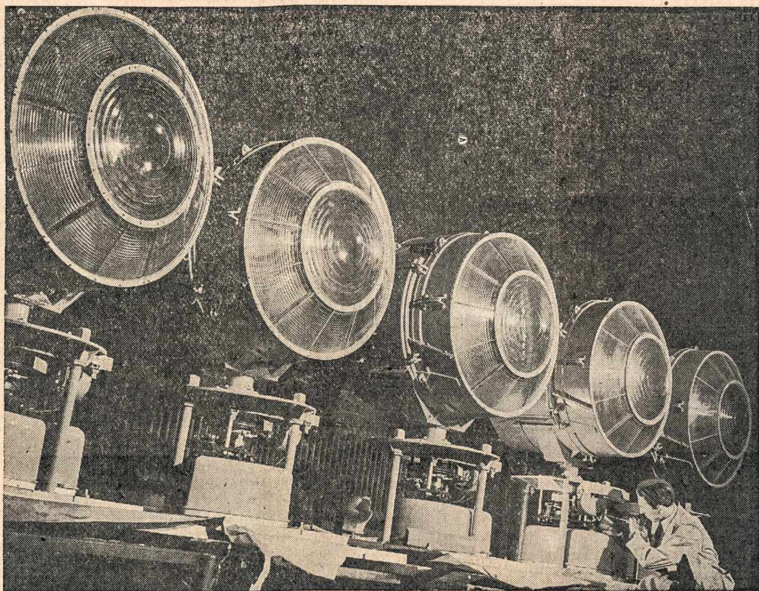
Milžiniški prožektorių veidrodžiai, kurie bus įtaisyti aukštumose, kad pasekus galimą prieš naktinį puolimą. Jie turi 36 inčių dvigubą veidrodį ir yra gaminami Cleveland Westinghouse dirbtuvėse.
