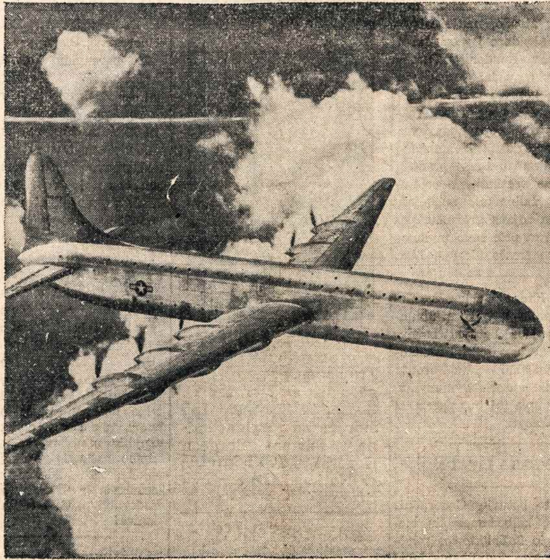
Šis lėktuvas tai naujas militaris transportinis Vultee's XC-99 skrenda išbandymo kelioj su 245,000 svarų kroviniu ir 13-ka žmonių įgulos. Jis pasirodė virš San Diego miesto ir yra vėliausias modelis išleistas po karo.
