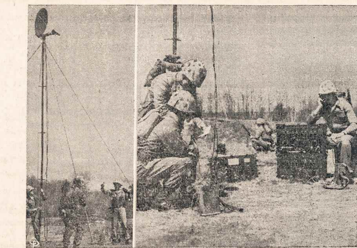
MARINŲ DALINYS (kairėje) netoli Waltham, Mass., stato 20 bėdų bokštą ir reflektorių, kuris naudojamas radijo ryšiams lauke. Dešinėje kareiviai prie radijo aparatu, kurių bangos yra labai trumpos ir veikia 40 mylių aplink. Šie aparatai pagaminti specialiai tam tikslui, kad galėtų palaikyti ryšį tarp kariuomenės dalinių, jeigu jos būtų atskirtos priešų.
