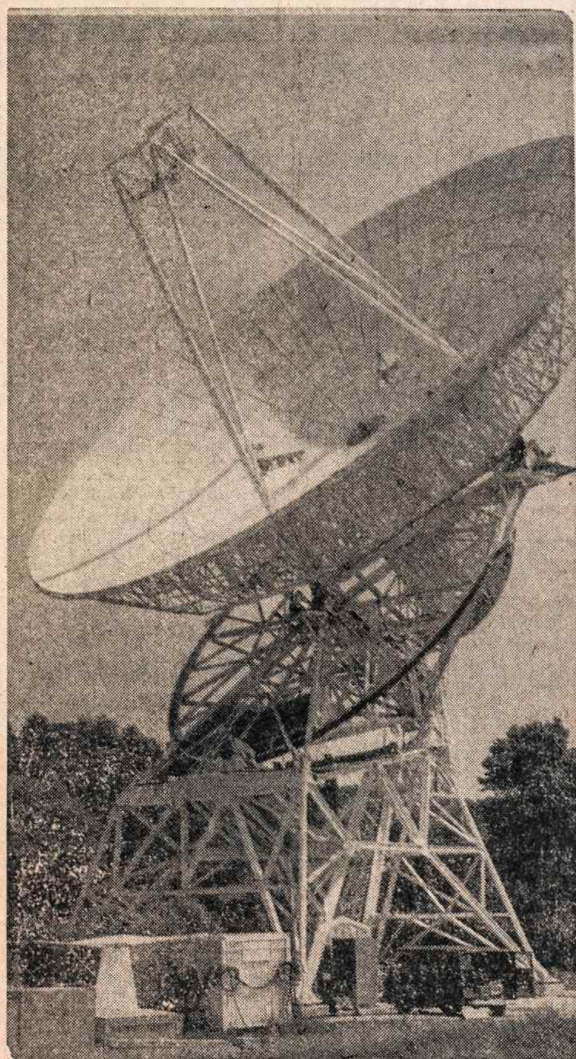
Ausys nukreiptos į visatą. Šios milžiniškos „lėkštės“ diametras 85 pėdos. Ji pagauna garsus, ateinančius iš žvaigždžių. Anglai turi 3 kartus didesnę „lėkštę“ — radijo teleskopą Jodrell Bank.
