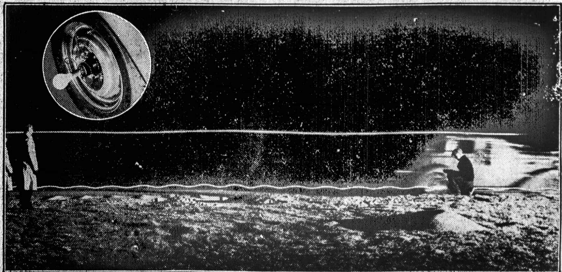
Fotografinė nuotrauka vaizdžiai parodo kaip sėkmingai veikia Chevrolet "knee action". Įrengtas su dviem lemputėmis automobilis—viena ant automobilio stogo, o kita—fate, važiuoja duobėtu keliu. Bet kaip rodo nuotrauka, nors ratai ir šokinėja, bet dėl "knee action", pats automobilis bėga lygiai, nē kiek nepsijudindamas, tarsi važiuotų labai lygiu keliu.
