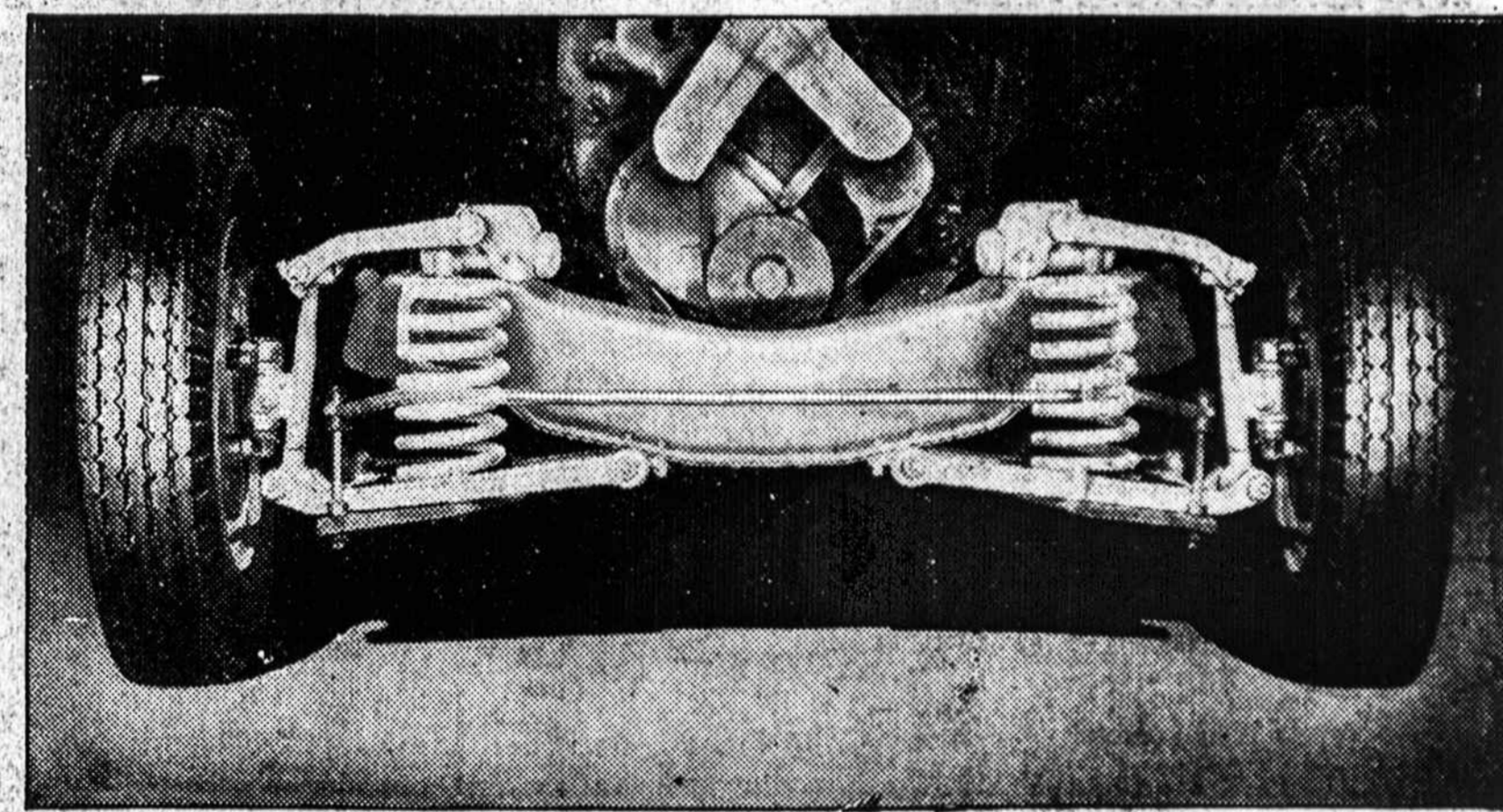
OLDSMOBILE "KNEE ACTION".—Nepaprastai patogų važiavimą ir lengvą vairavimą, taipjau ir didesnę saugumą suteikia pagerintas "knee action" 1938 metų Oldsmobile automobilis.
