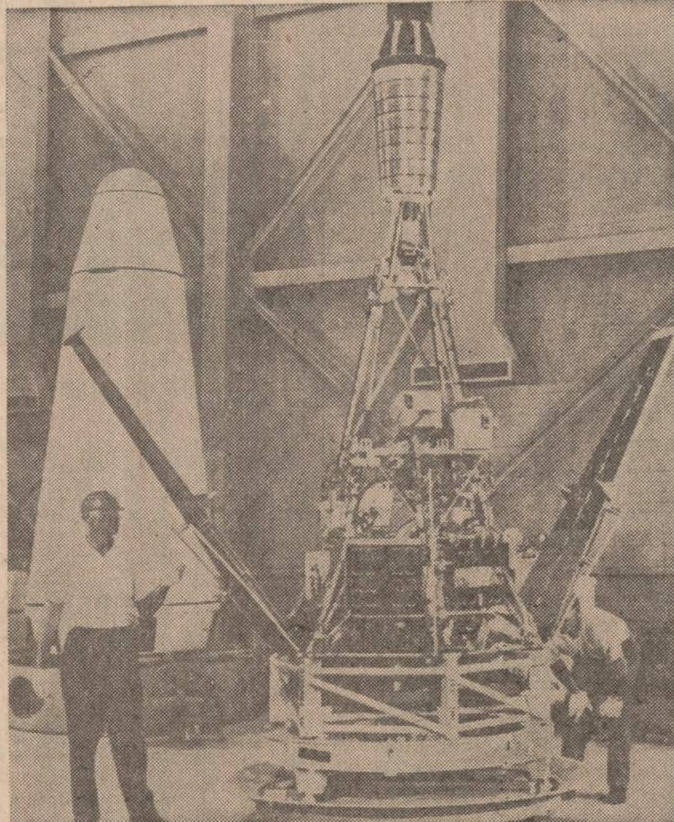
Projektuojamas erdvės tyrimo prietaisas. Čia Ranger 1, pirmasis iš erdvės laivų serijos, kuris bus JAV sviestas į erdvę ir eventualiai panaudotas labai jautriems prietaisams nugarinti mėnulį. Manoma, kad pirmą kartą šis 675 svarų prietaisas priartės prie mėnulio iki 35,000 mylių. Mokslininkai tikisi, kad jis praskins kelis atšities šūvius, kuriais bus nugarinti prietaisai ir mėnulį. Čia techniškai tikrina satelitą. Cape Canaveral, Fla.
