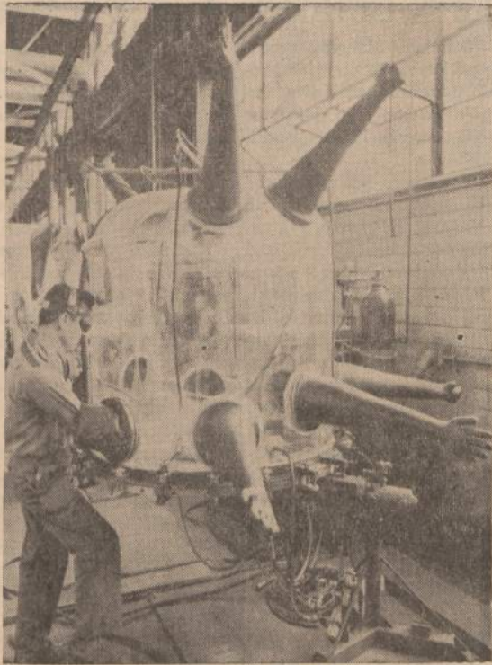
McDonnell įmonėje (St. Louis, Mo.) yra gaminama nauja Geminė erdvės kapsulė dviem žmonėm. McDonnell įmonėje buvo pagaminta ir Mercury kapsulė (vienam žmogui), kuri apsisuko aplink žemę.
