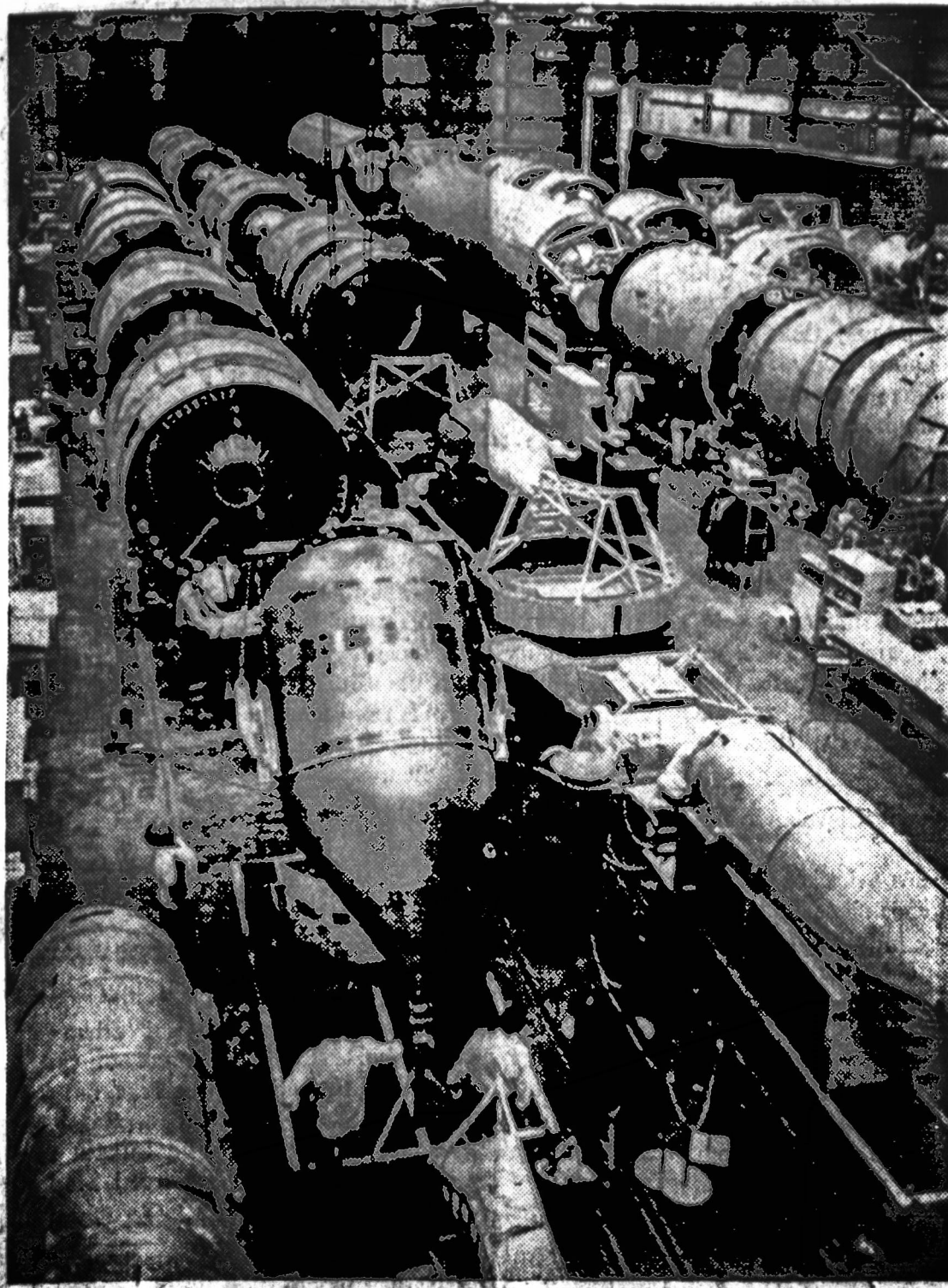
Titan 3, deguonių tankas, Davaur, Aisturvyje, Iklainas, raketos. Šis ir kitantimo pagamintus tankus turi 12 pėdų ilgio ir 5 pėdų diametrą.
