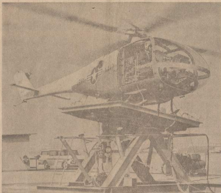
Helikopteris pastatytas ant besikraipiančios platformos, kad laivu plaukiantieji lakūnai priprastų lipti į helikopterį bet kurioje kryptyje.
