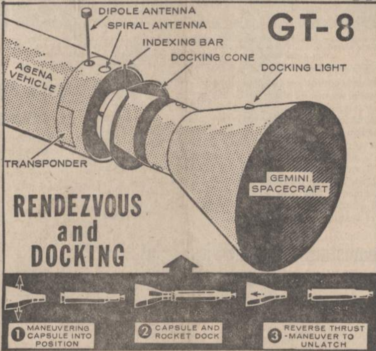
Paveikslas rodo, kaip Gemini raketa susijungs su Agena ir kaip ji išsijungs. Tai bus pats sunkiausias astronautų manevras erdveje.
