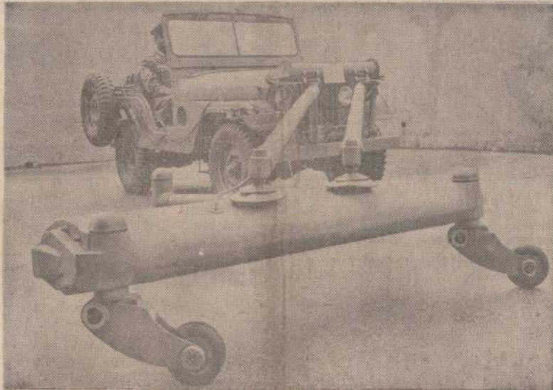
Vietnamo fronto linijomis važinėjantieji džipai gavo naują prietaisą komunistų pakastoms minoms surasti. Paveiksle matomas prietaisas suranda miną ir momentaliai išjungia motora. Automobilis nevažiuoja ant minos ir apsaugo karius. Minų ieškotojas gali apžiūrėti kelį 10 mylių į valandą greičiu.
