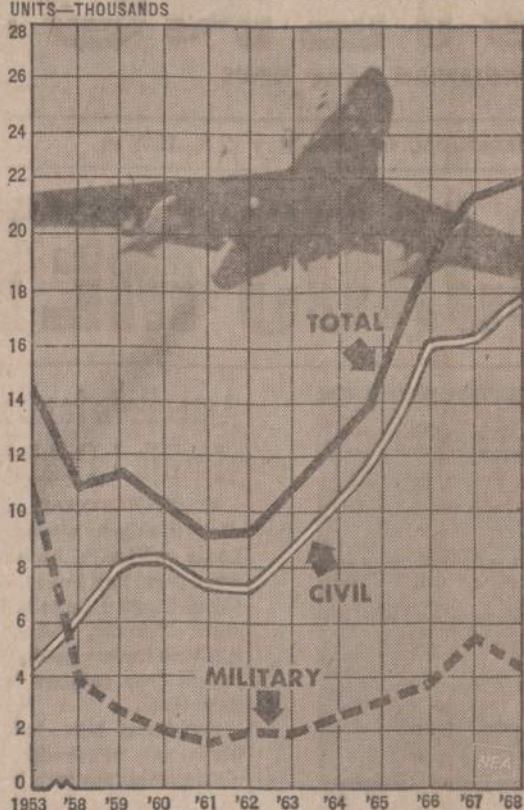
Praeitais metais lėktuvų gamyba Amerikoje buvo sumažėjusi, bet pirmieji šių metų mėnesiai pakeitė vaizdą. Šiais metais sumažėjo karo lėktuvų gamyba, bet keleivinių lėktuvų gamyba padidėjo. Manoma, kad šiais metais lėktuvų gamyba dar didės, nes yra daug naujų užsakymų.
