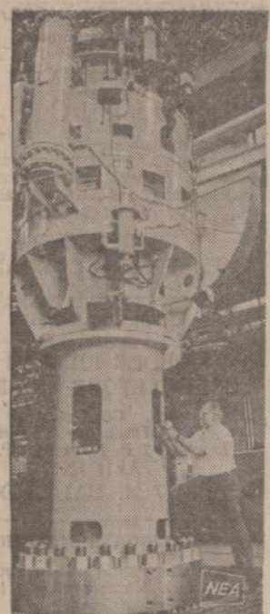
Paveiksle matoma pompa yra 28 pė-dų aukščio ir sveria 192,000 svarų. Ji pastatyta Cheswick, Pa. miestelyje, kur Westingouse bendrovė gamina atominę energiją. Inžinieriai apskai-čiavo, kad kiekviena minutė šiai pom-pai teks išmesti 88,500 galonų van-dens.
