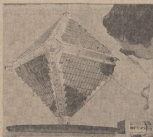
Paveiksle matomas prietaisas erdvėje gali rinkti elektronus ir protonus. Šiomis dienomis jis bus iškeltas į erdvę, rinks atomo dalelytes ir praneš žemėn, kaip jam sekasi.
