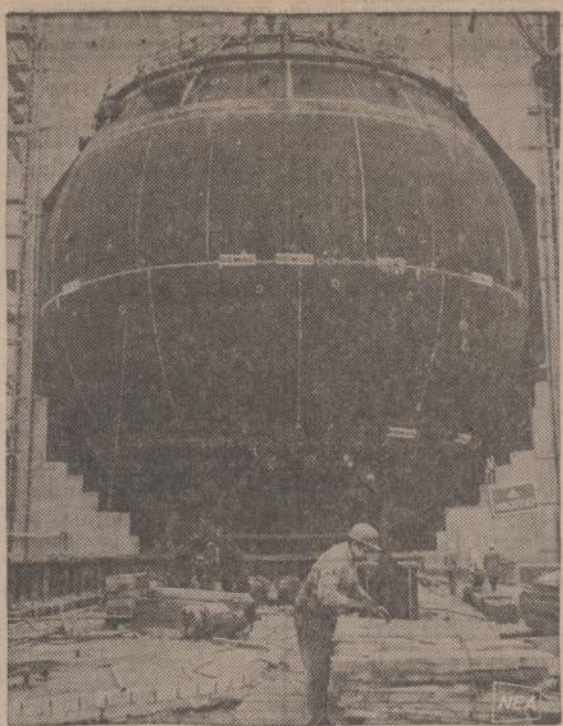
Wuergassen miestelyje vokiečiai pasistatė dirbtuve atomui skaldyti. Statyba šioje vietoje buvo atstatoma namas visoms dirbtuvoms ir tuo pačiu metu buvo statomas prietaisas atomui skaldyti. Kai namas buvo baigtas statyti, tai vežiam mašina atomui skaldyti buvo įstumta į savo vietą pro sienoje paliktą plyšį. Vokiečiai sutaupe daug reikalingo laiko, nors mašinos į savo vietą įstūmimas buvo gana lėtas.
