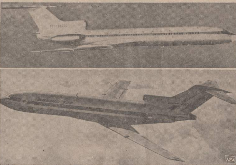
Viršuje naujas sovietų keleivinis sprausminis lėktuvas TU-154. Jis gali nešti 160 keleivių. Šis lėktuvas pasirodė aplankyti 46 valstijas, įskaitant ir JAV. Apačioje matoma nauja JAV lėktuva Boeing 727. Jis gali nešti 114 keleivių. Amerikiečių pastatytas lėktuvas truputį mažesnis, jam lengviau nusileisti ir pakilti mažesniuose aerodromuose.
