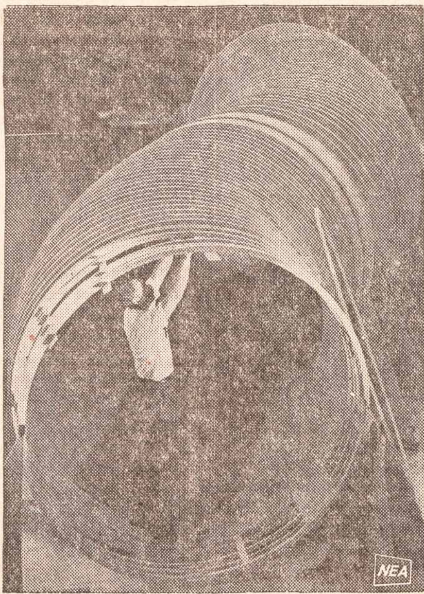
Naujai Lockheed bendrovės statomam trijų motory sprausniam lėktuvui reikalingas didelis vamzdis orui įtraukti. Paveiksle statomas toks vamzdis bus 30 pėdų ilgio ir 7 pėdų pločio. Iš lėktuvo viršaus traukiamas oras šiuo vamzdiu eis į užpakalyje esantį motora.
