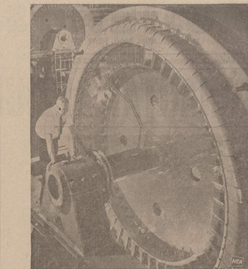
Allis - Chalmers elektros bendrovė pagamino šį 3,000 arklio jėgų motorą, kuris Arizonos kasykloje vėrys vario rūdai išskirti iš akmenų malūna. Tokių malūnų kasykla turės 14. Motoras pagamintas Wisconsin.
