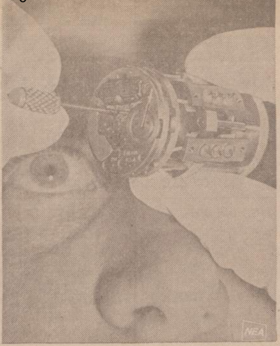
Erdvėlaivys, kuris skris į Mėnulį, yra daug įvairiausių aparatų. Čia matomas Bufova bendrovės gamintas instrumentas, kuris liks Mėnulyje ir kitiems aparatams duos signalus, kada pradėti kokį veiksmą.
