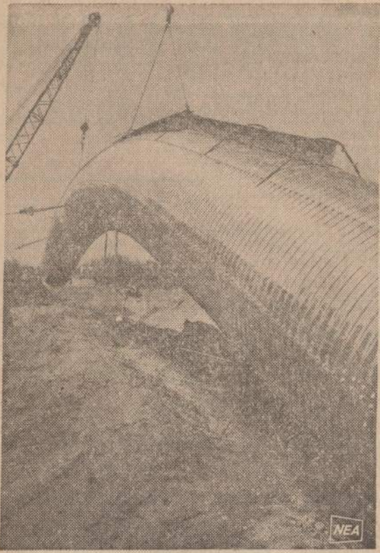
Irigacijos vamzdžių tiesimas labai pagreitėjo su naujais Armo Multi-Plate vamzdžiais. Keltuvus pakelia 180 pėdų ilgumo ir 8 pėdų diametro vamzdžio gala ir padeda jį į tam tikslui įkaste griovį. Nereikia daug darbininkų ir darbas daug švaresnis.
