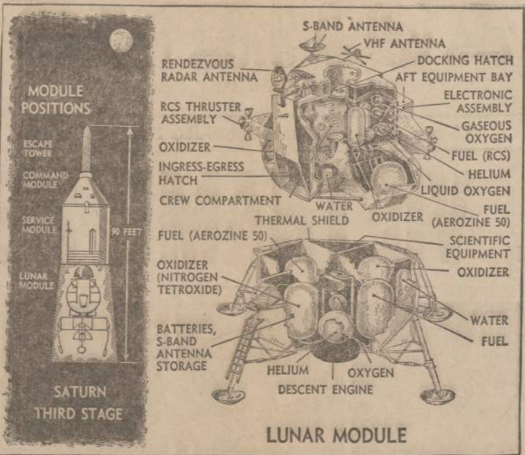
Sudėtinga Mėnulio erdvėlaivio aparatūra parodoma dešinėje, o kairėje matoma trečioji Saturno raketos dalis, susidedanti iš Apollo erdvėlaivio ir Mėnulio nusileidimo laivo-Voro, kurio "kojas" astronautai paliks Mėnulyje, pasikeldami sugrįžimui.
