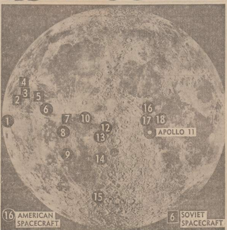
Nors astronautai Armstrongas ir Aldrinas yra arba bus pirmieji žmonės Mėnulyje, tačiau žmonių pasiūtų įvairių laivų Mėnulio paviršiuje jau nemažai. Fotografijoje pažymėtos vietos, kur nusileido ar sudūzo amerikiečių ar sovietų pasiūti erdvėlaiviai: Orbiter, Luna, Surveyor, Ranger pavadinimais. Amerika pasiuntė 16, sovietai 6.
