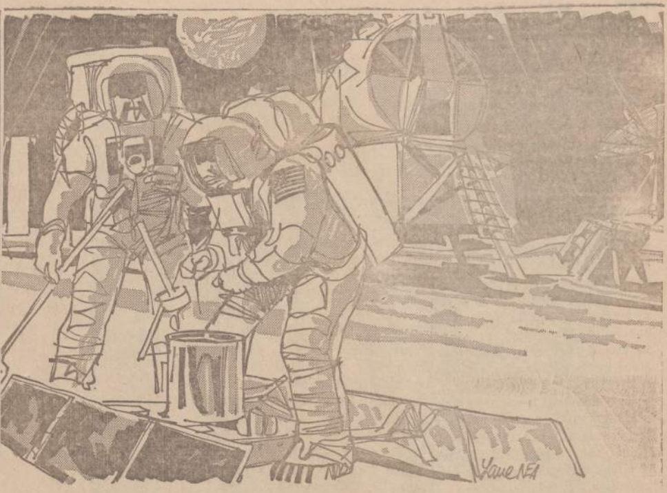
Astronautai mėnulyje turės atlikti visą eilę darbų: išvynioti lakštą alumino, kuris turės pagauti ten esančias dujas, bus matuojamas solarinis vėjas. Antenos pagaus žemės signalus, kurie padės išmatuoti atstumą tarp planetų centimetro tikslumu.
