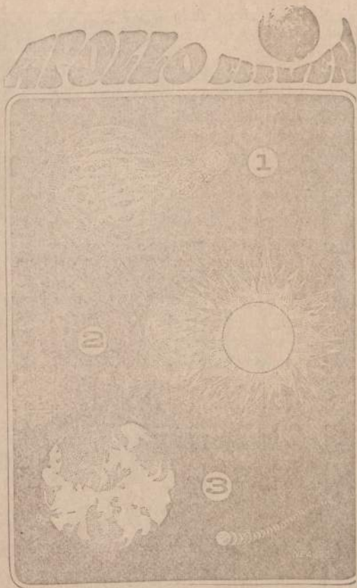
Amerikos astronautų nusileidimas ant Mėnulio gal padės išspręsti klausimą, iš kur Mėnulis atsirado. Pagrindines yra trys teorijos. Pirmą sako, kad Mėnulis yra Žemės dalis, atsikilęs prieš milijonus metų dėl nežinomo priežasties. Antra teorija — Mėnulis susidarė tuo pačiu metu kaip Žemė iš solarinių dulkių ir dujų, o trečia teorija tvirtina, kad Mėnulis atklydo iš tolimų erdvių ir liko priiritas prie Žemės jos traukos jėgos.
