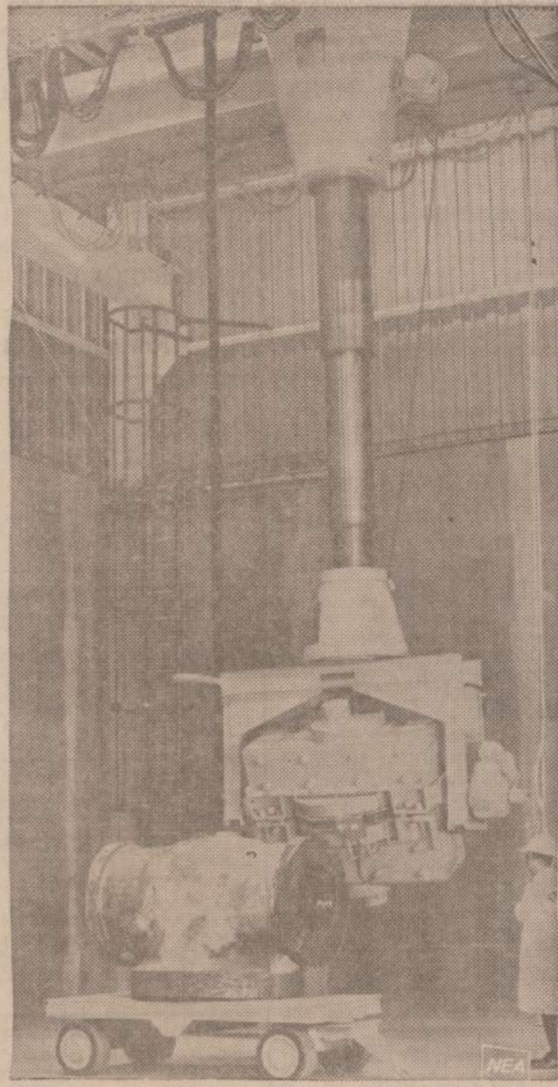
Kalifornijoje yra mižiniškas rentgeno spindulių aparatas, kuris pa- tikrina metalo lydinius. Aparatas kainavo 25 milijonus dolerių. Jis pastebi ir praneša apie lydinių netobulumus ir silpnas vietas.
