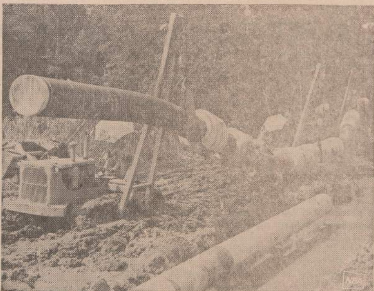
Louisianos raistynuose tiesiama natūralių dujų vamzdžių linija turi cementinius "inkarus", kurie laiko vamzdžius žemėje. Du traktoriai tiesia 30 colių vamzdžius. Jų bendras ilgis sudarys visame krašte 860,000 mylių.
