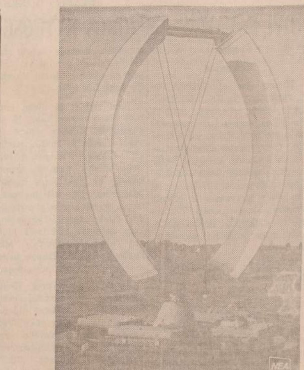
Laivas - robotas, sugalvotas ir pastatytas RCA inžinierių, pats be igulos, valdomas radijo signalais, gali nuplaukti su elektroniniais prietaisais į bet kurį jūrą ir be inkaro plaukiooti vietoje, kol signalai iš pasius kitur. Apatyje tokie laivai bus naudojami ero tyrimams, šnipinėjimui ir kitiems tikslams. Laivas turi pastovias bures ir automatinus irklus.
