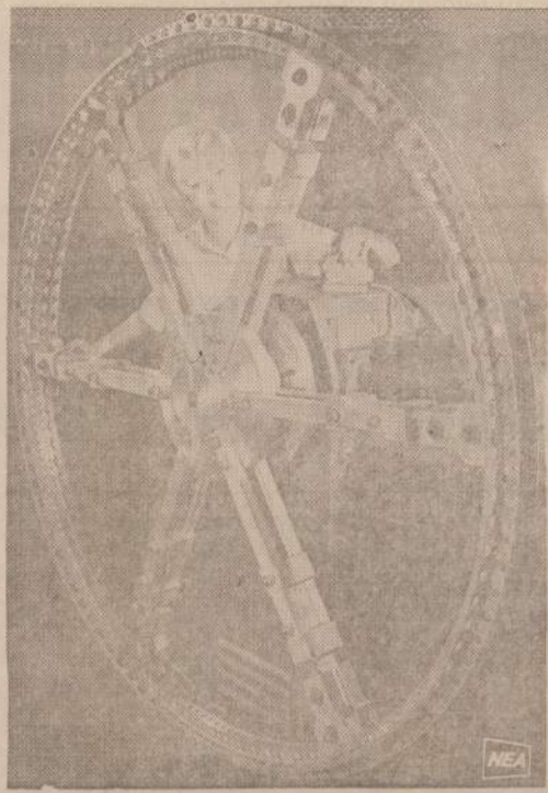
Šis ratas, pagamintas Princetono universiteto fizikos laboratorijoje, teorškai turėtų erdvėje laisvai palaikomas savo paties gamtinamos magnetinės jėgos. Rato krašte yra 12 mylių ilgumo nobiumo kaspinas, kuris pamoktas į skysta helijū praleidžia elektros srovę ir gamina magnetinį lauką. Už rato pastatyta mergina skirta šios neįdomios fotografijos pagražinimui.
