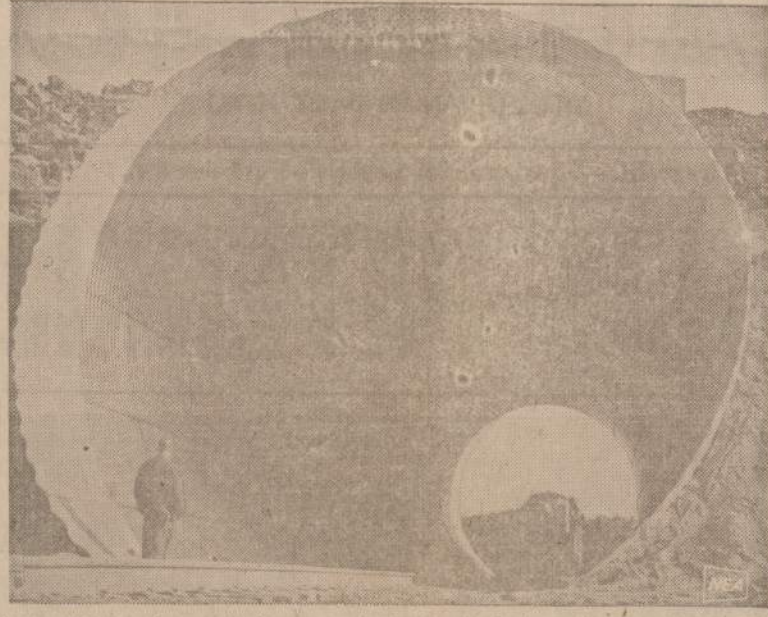
Palmer, Michigan viename fabrike yra pastatytas tunelis, kuriuo važinėja traukiniai. Viršuje eina kelias. Tunelio pagrinde 190 pėdų ilgumo ir 30 pėdų diametro metalinis vamzdis. Jis svėrie 200 tonų. Tokius tunelius greičiau ir pigiau galima pastatyti, negu iš plytų mūrijant.
