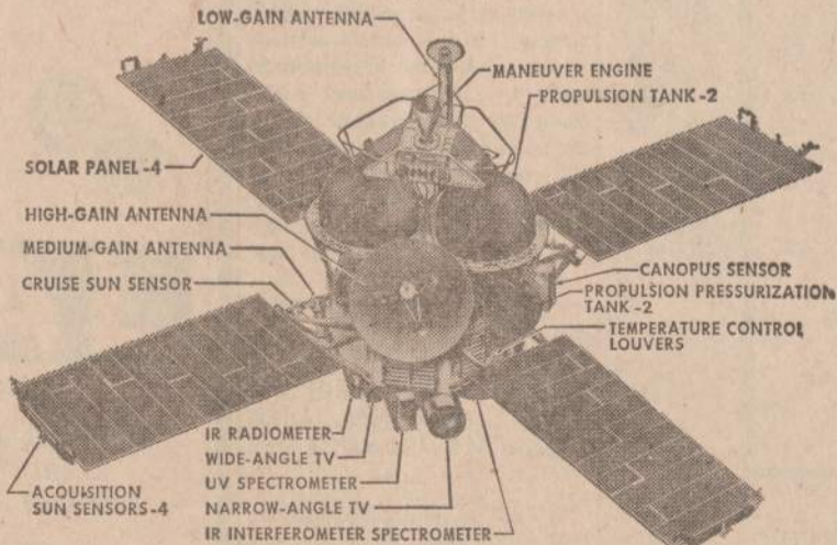
Šitokie Mariner erdvėlaiviai bus siunčiami 1971 metais į Marso planetos apylinkes.
