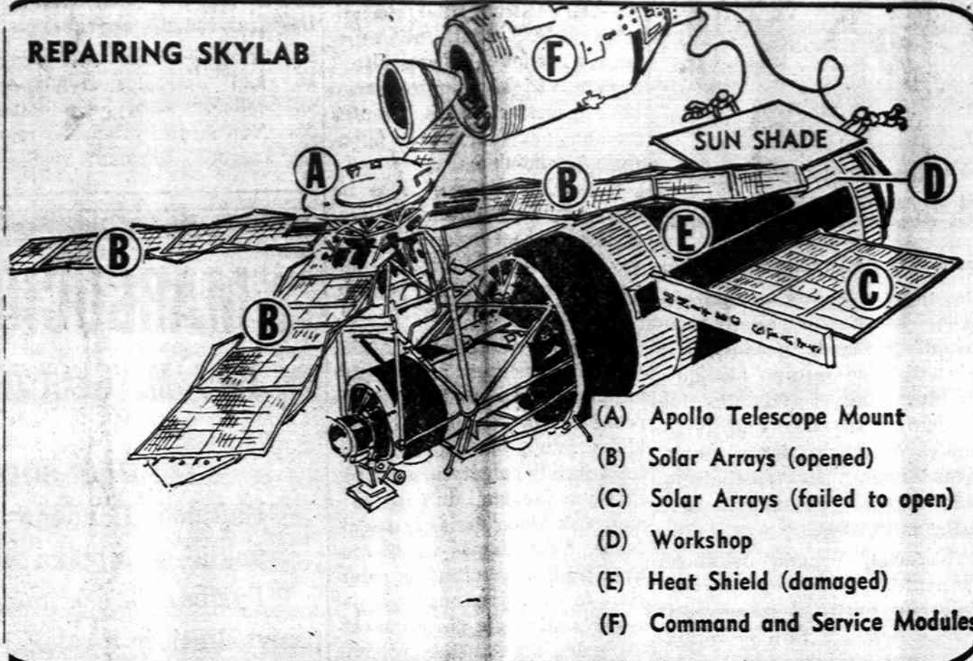
Skylab erdvės stoties piešinys. Dešinėje, viršų parodoma, kaip astronautai bandys pakeisti nuplėštą saulės spindulių izoliaciją — maršką, kuri nepraleistų saulės karštų spindulių.
